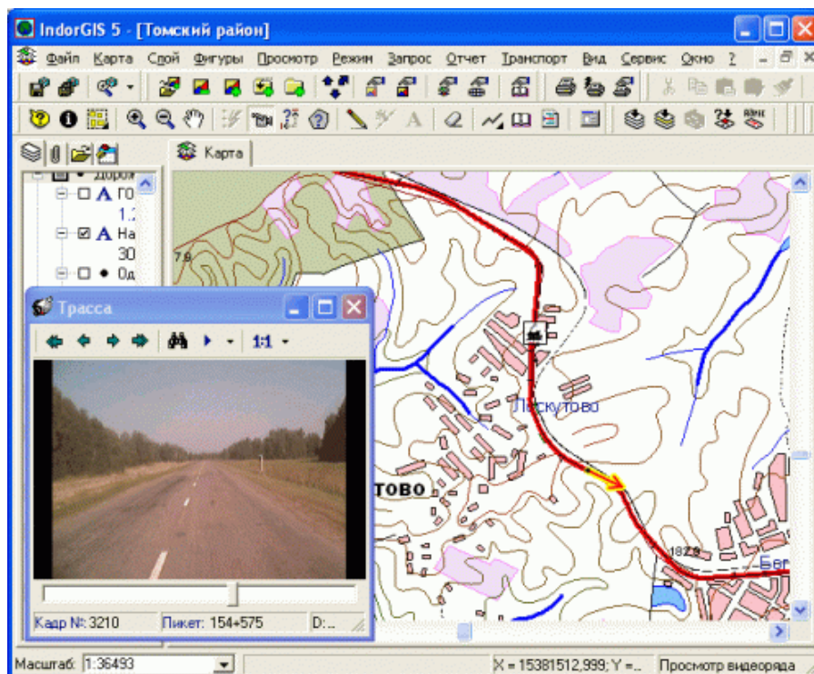
Рис. 5. ГИС-платформа IndorGIS
