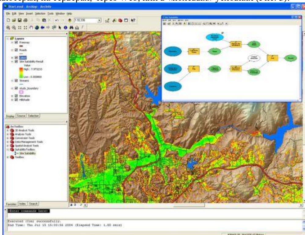
Рис.3. ГИС-платформа ArcGIS 9
