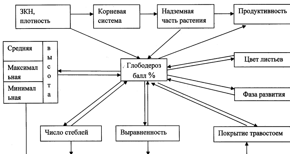
Рис. 1. Схема логической модели взаимодействия популяций ЗКН и растения-хозяина картофеля и структуры модулей показателей, определяющих развитие глободероза картофеля
