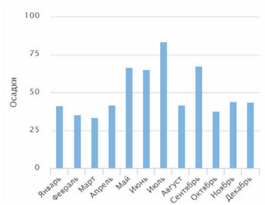
Рис. 3. Среднемесячное количество осадков в Калужской области [Fig. 3. Average monthly precipitation in the Kaluga region]
